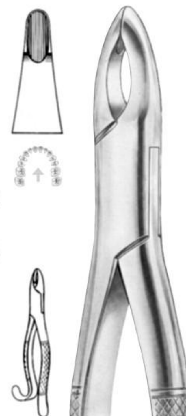
KTS10831 # 213 obere Schneide- und Eckzähne upper centrals and canines incisives et canines supérieures incisivos y caninos superiores
