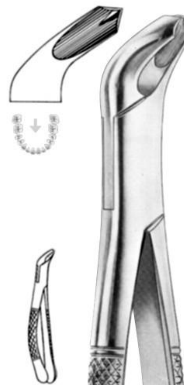
KTS10832 # 217 untere Molaren lower molars molaires inférieures molares inferiores
