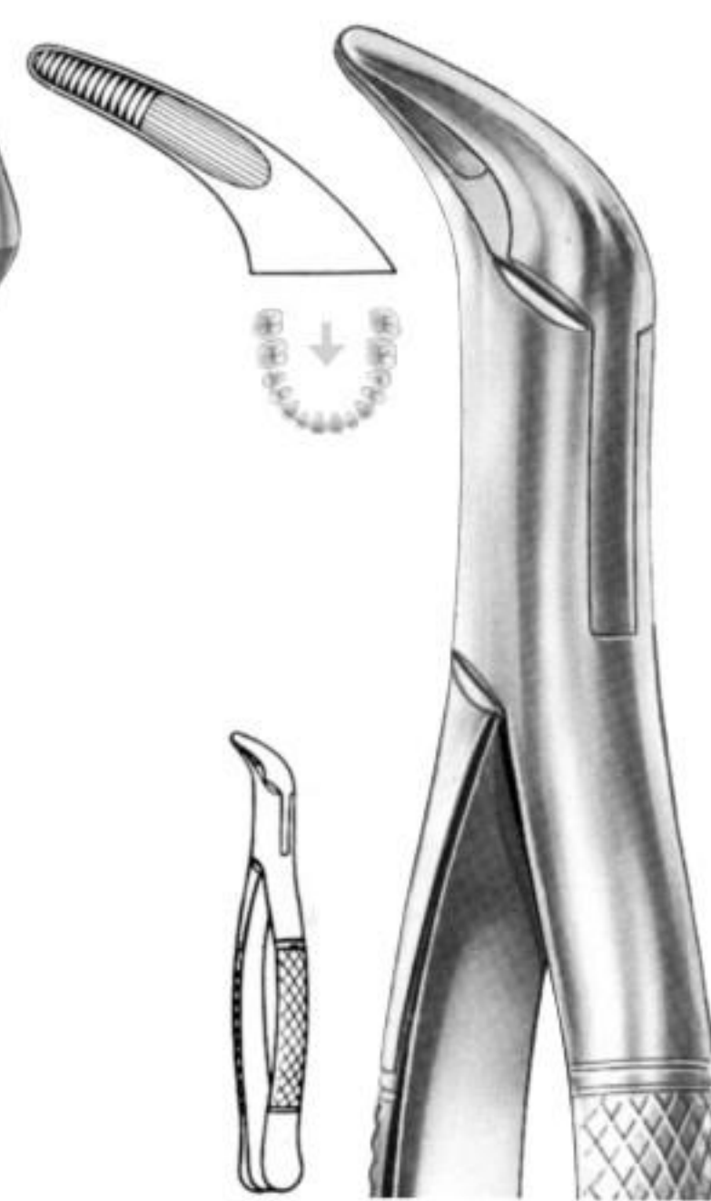
KTS10804 # 36 untere zähne, und wurzeln lower anteriors, and roots dents et racines, inférieures dientes y raíces inferiores
